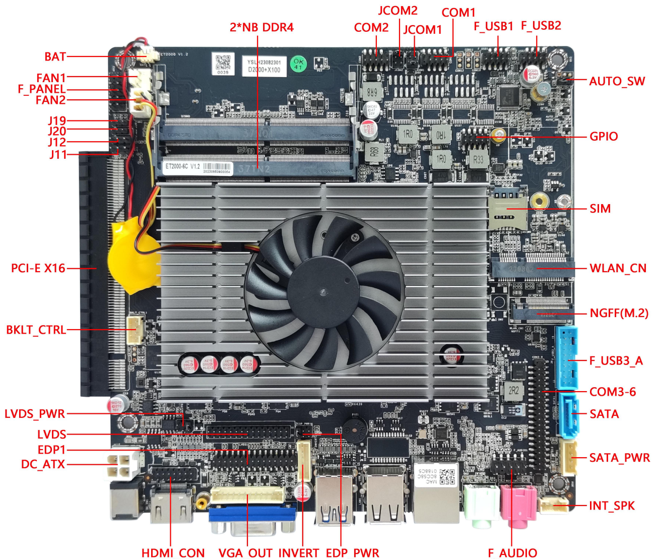
6COM 主板示意图 ↓
