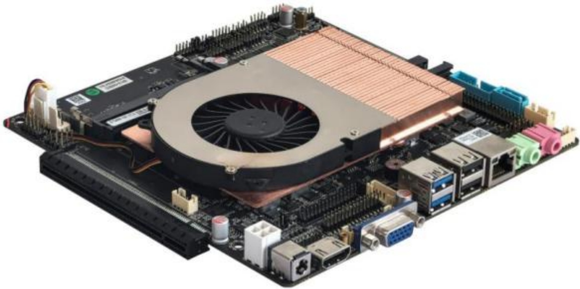
铜管散热器示意图 ↓
