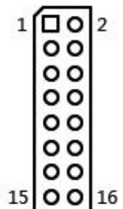
插针位号图
