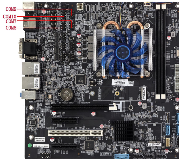
10COM 主板示意图 ↓
