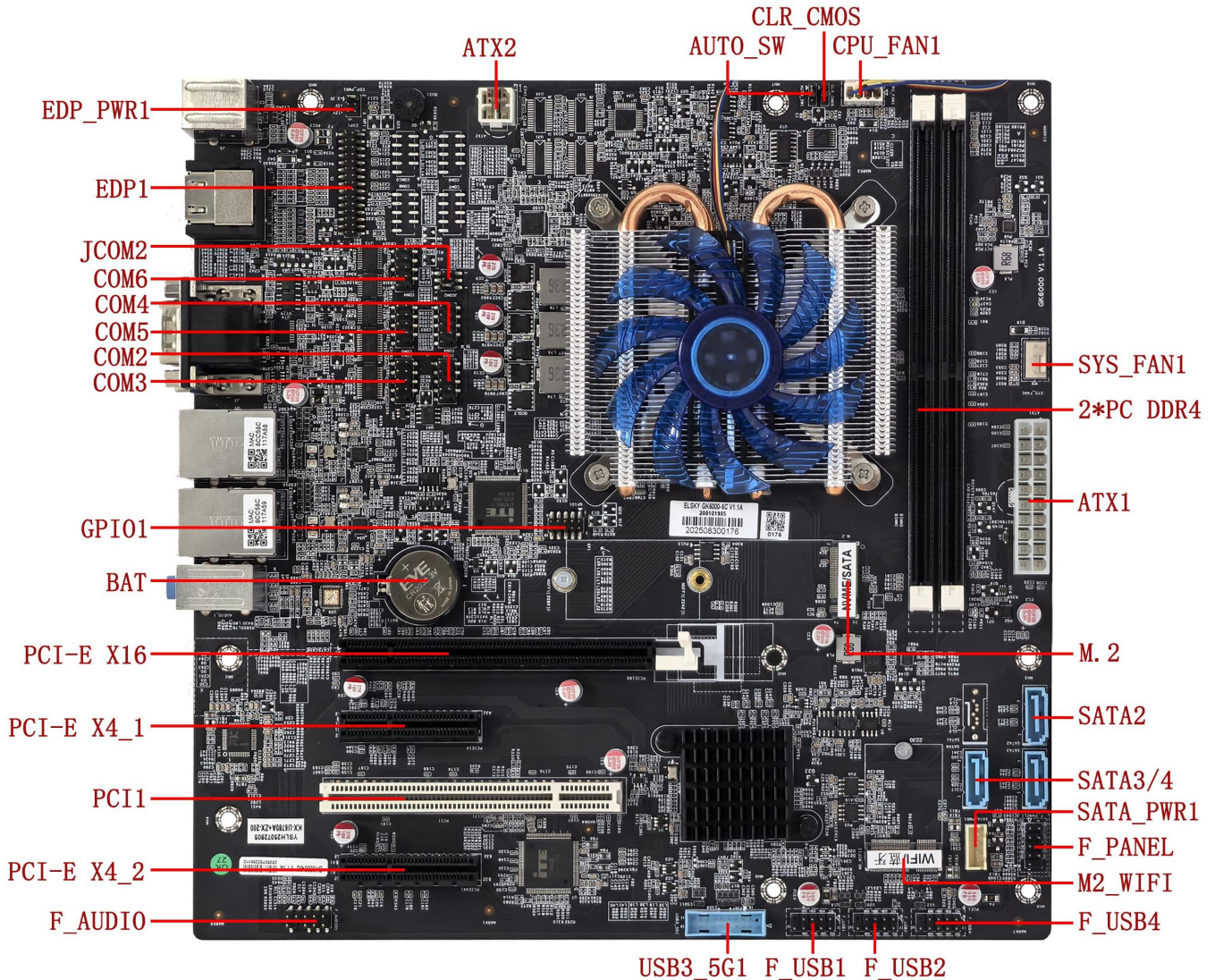
6C 主板示意图 ↓
