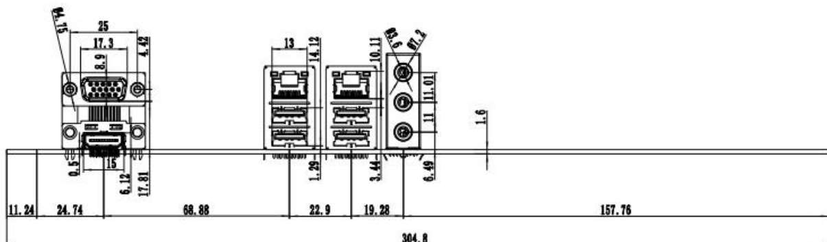
接口尺寸图↓
