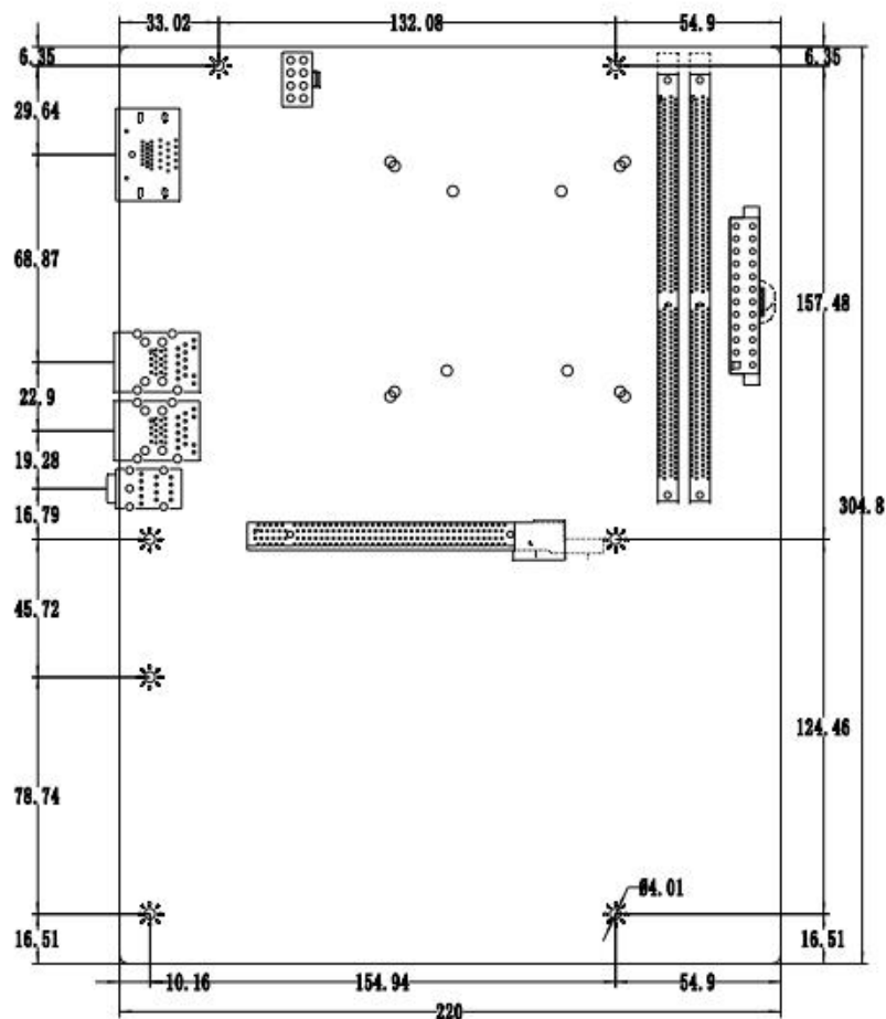
接口尺寸图↓
