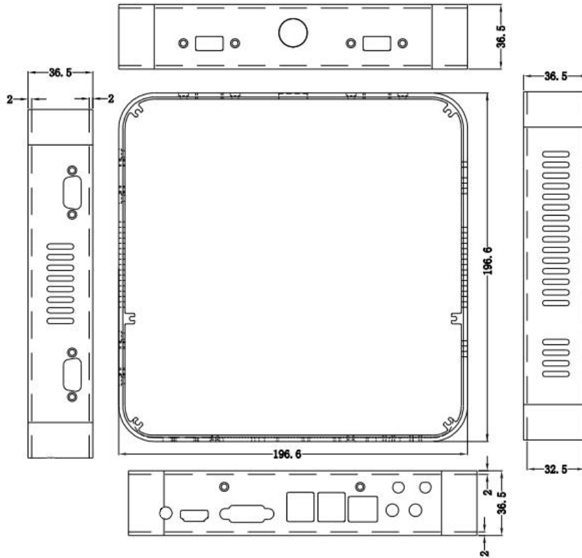
主机底部尺寸示意图 ↓
