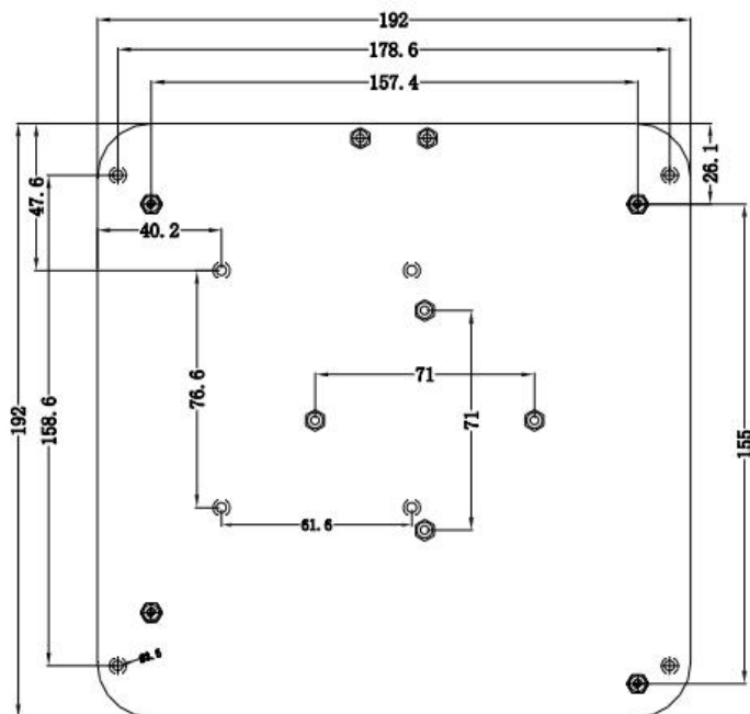
主机底部尺寸示意图 ↓
