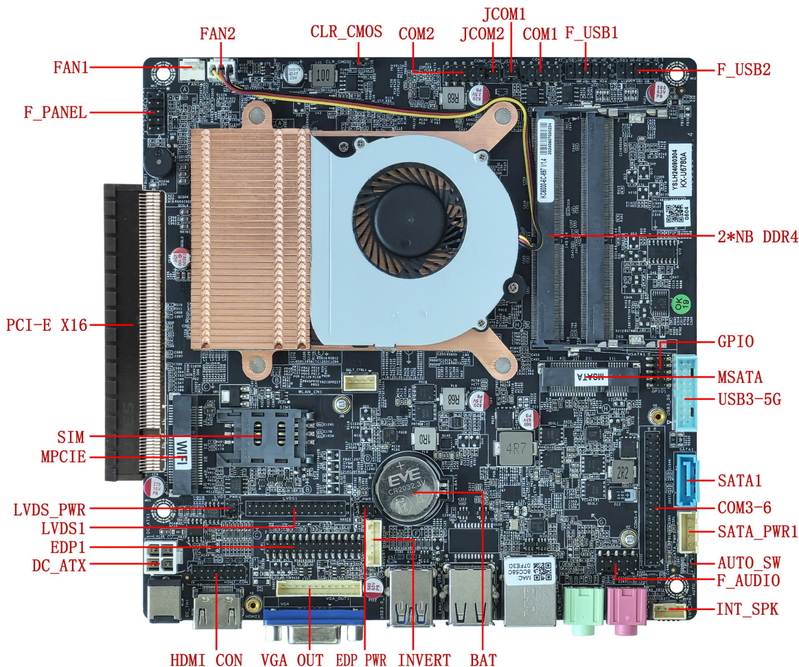
主板示意图 ↓
