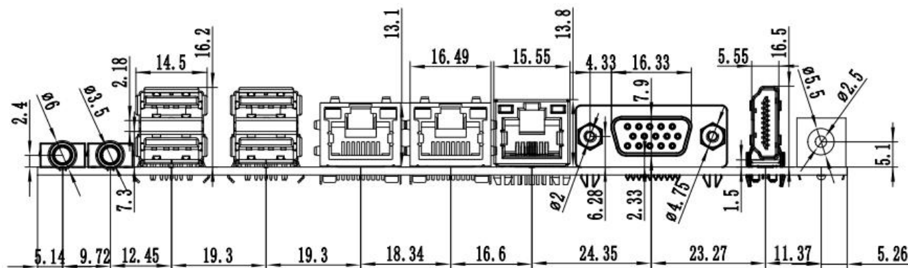
三网口尺寸
