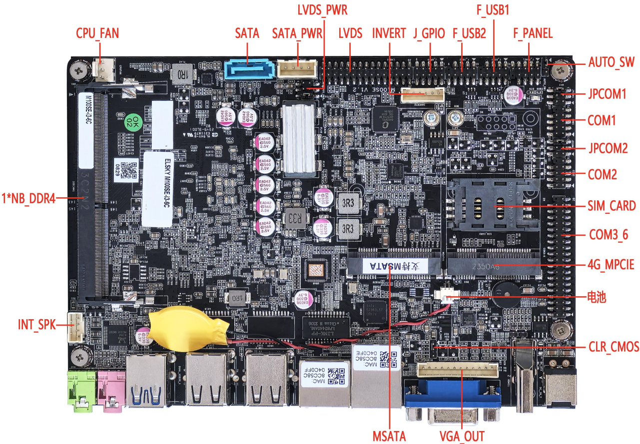
主板示意图 ↓
