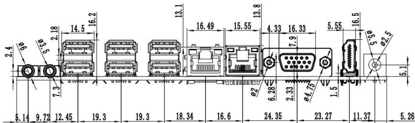
双网口尺寸
