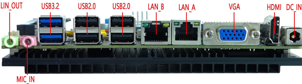
双网口主板接口示意图 ↓
