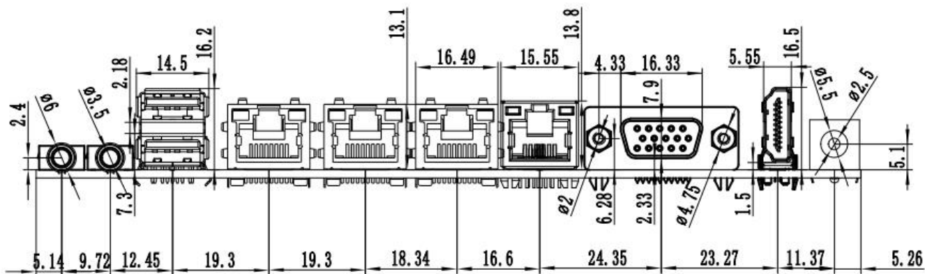
四网口尺寸
