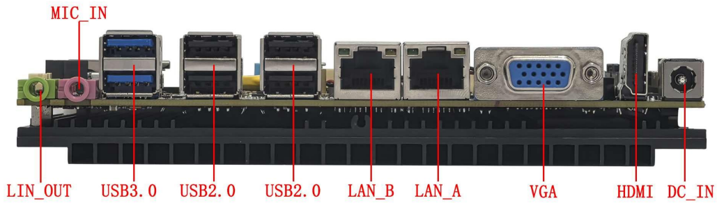
VGA+HDMI+双网 接口示意图 ↓
