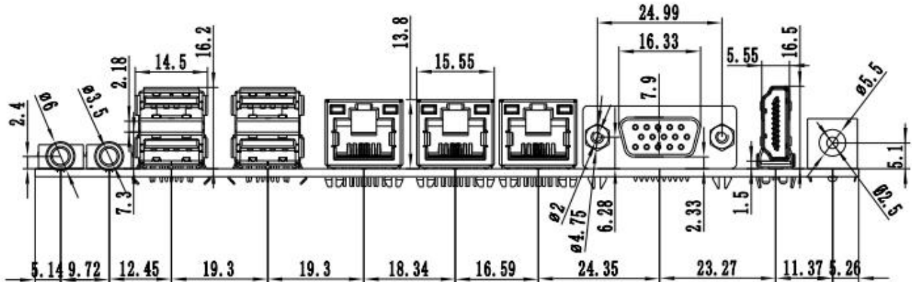
VGA+HDMI 三网口尺寸 (VGA 尺寸只适用于 v1.2 版本)
