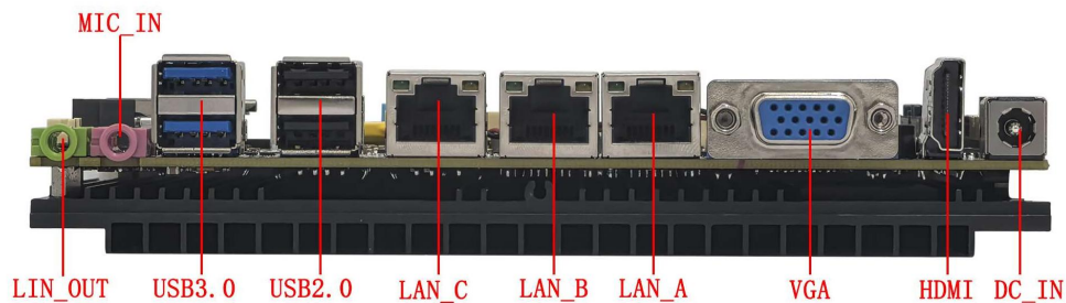
VGA+HDMI+三网 接口示意图 ↓
