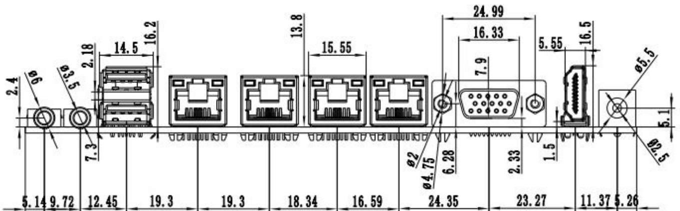
VGA+HDMI 四网口尺寸 (VGA 尺寸只适用于 v1.2 版本)
