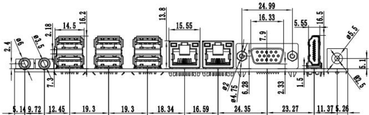
VGA+HDMI 双网口尺寸 (VGA 尺寸只适用于 v1.2 版本)
