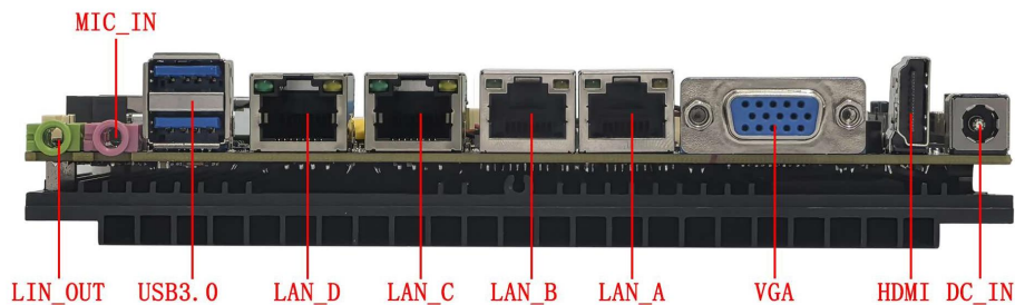
VGA+HDMI+四网 接口示意图 ↓
