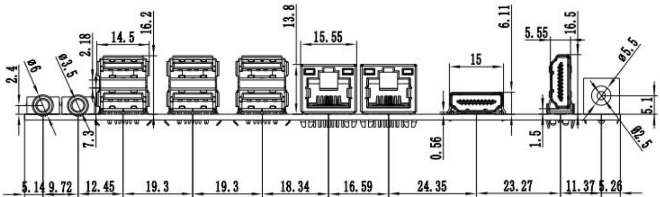
双 HDMI 双网口尺寸
